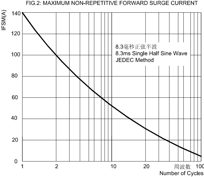
图2: 最大正向浪涌冲击耐受力
