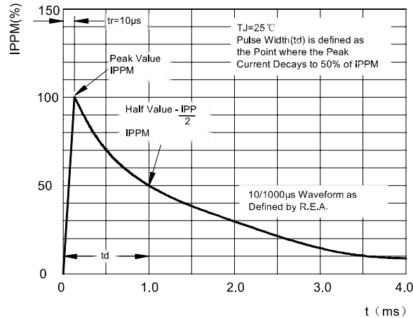
图3: 脉冲波形 FIG3: Pulse Waveform
