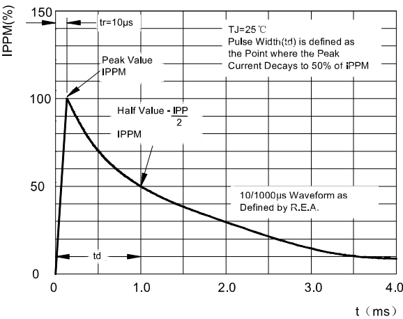
图5：最大不重复浪涌电流
