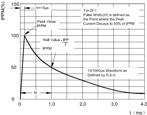
图3：脉冲波形 FIG3: Pulse Waveform
